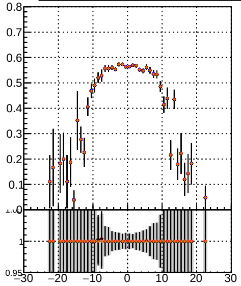
Efficiency vs. sim PV z —●— DQM TT MS —●— DQM TT MS detT —●— DQM TT MS detT-dpdq —●— DQM TT MS detT-chi2
