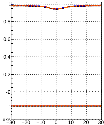
Fake rate vs v DOM TT MS det0 det01 det09
