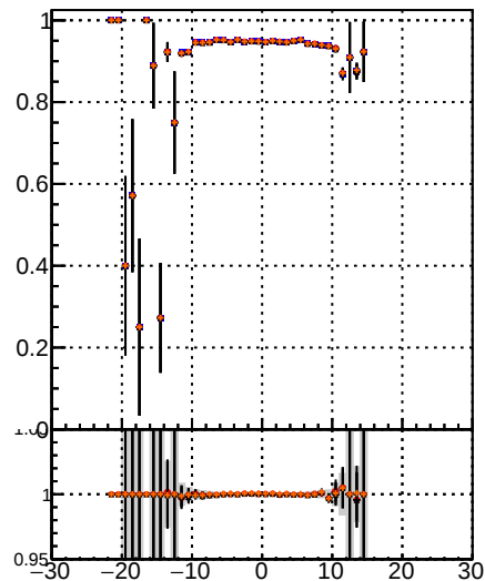
Fake rate vs v DOM TT MS det0 DOM TT MS det01 DOM TT MS det09
