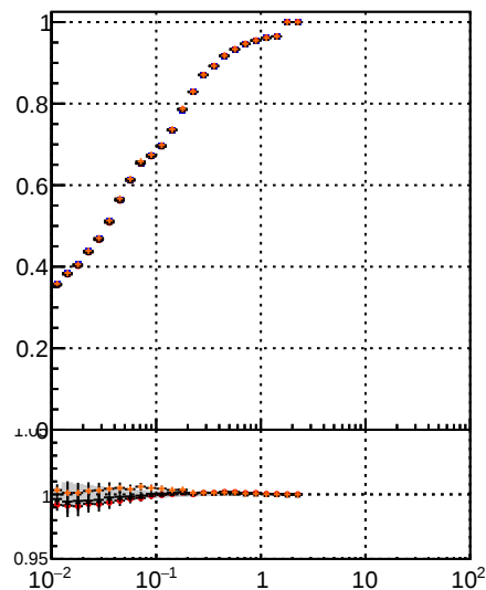
Fake rate vs \sqrt{s} Model TT MS detQ detQ1 detQ9 DOM TT MS detQ detQ1 detQ9 DOM TT MS detQ detQ1 detQ9 DOM TT MS detQ detQ1 detQ9
