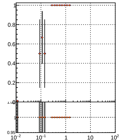
Fake rate vs v DOM MS det0 det01 det09
