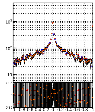
—●— DQM TT MS-det00 —●— DQM TT MS-det01 —●— DQM TT MS-det09
