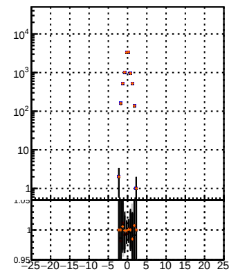
—●— DQM TT MS-det00 —●— DQM TT MS-det01 —●— DQM TT MS-det09
