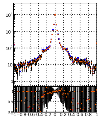
N of reco track vs dxy(PV) MS-det01 MS-det09
