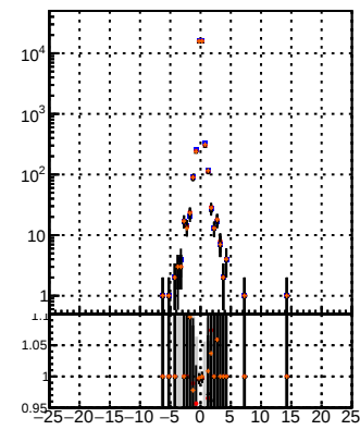
N of reco track vs dxy(PV) MS-det01 MS-det09
