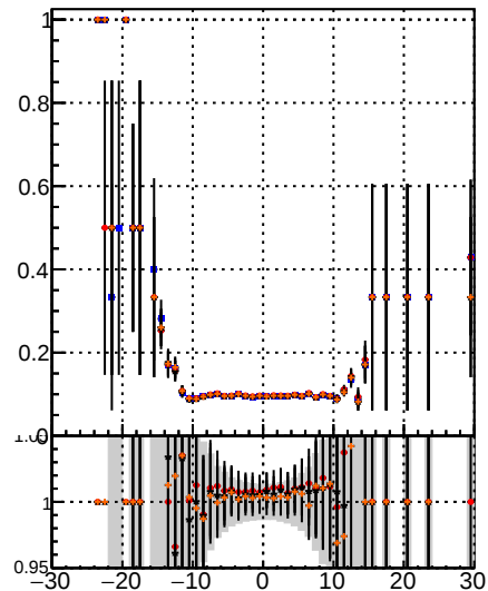
Fake rate vs d DQM MS data DQM MS data
