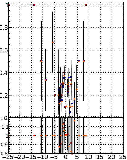
Fake rate vs d DQM MS data DQM MS data
