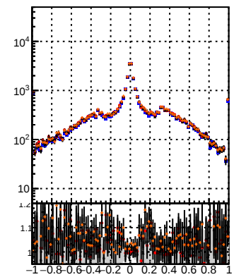
— DQM — MS — MS-det09 — DQM — MS — MS-det09 N of reco track vs dxy(PV)
