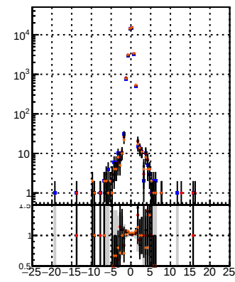
— DQM — MS — MS-det09 — DQM — MS — MS-det09 N of reco track vs dxy(PV)
