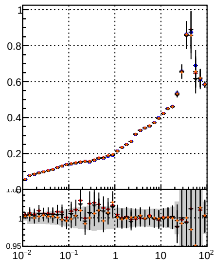
Fake rate vs \nu —■— DOM TT MS det0 —●— DOM TT MS det0 —▲— DOM TT MS det0 —×— DOM TT MS det0
