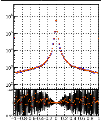
—●— DQM TT MS-det09 —●— DQM TT MS-det09 —●— DQM TT MS-det09
