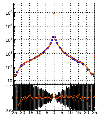
—●— DQM TT MS-det09 —●— DQM TT MS-det09 —●— DQM TT MS-det09
