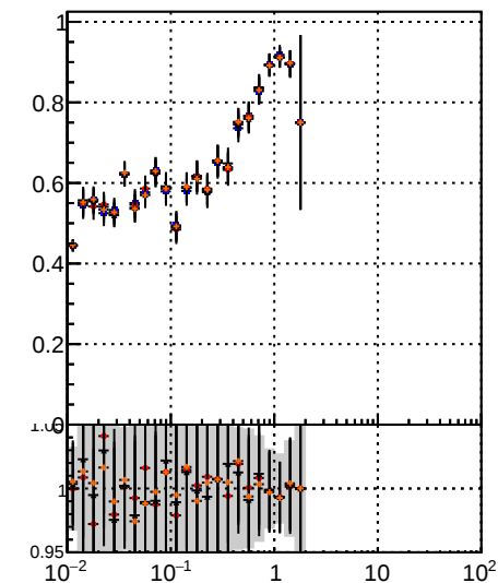
Fake rate vs \sqrt{s} —●— \sqrt{s} MS det0 —●— \sqrt{s} MS det01 —●— \sqrt{s} MS det09
