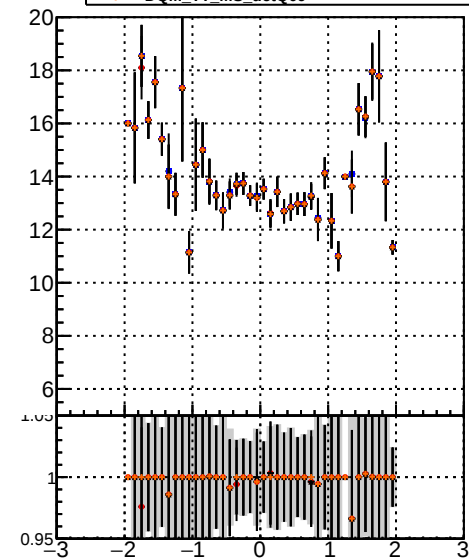
mean hit DQM TT MS DQM TT MS_detQ DQM TT MS_detQ1 DQM TT MS_detQ09
