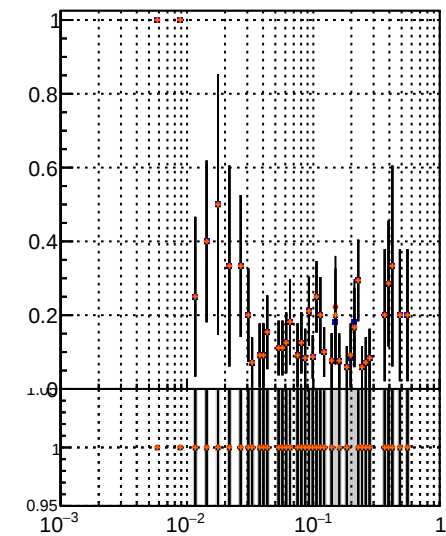
Fake rate vs DOM TT MS det0 det01 det09
