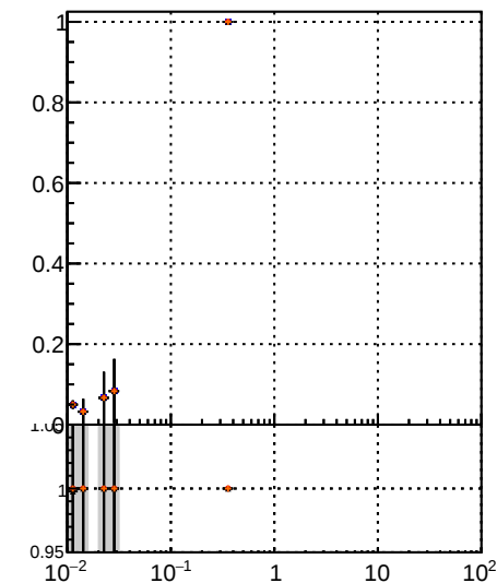
Fake rate vs v DOM TT MS det0 DOM TT MS det01 DOM TT MS det09
