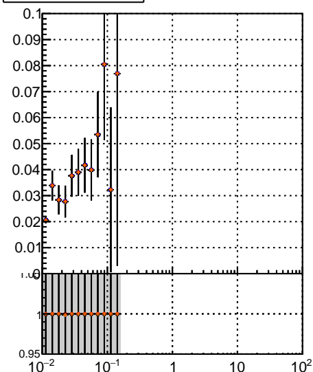
Fake rate vs \sqrt{s} —●— DQM TT M6 detQ —●— DQM TT M6 detQ1 —●— DQM TT M6 detQ9
