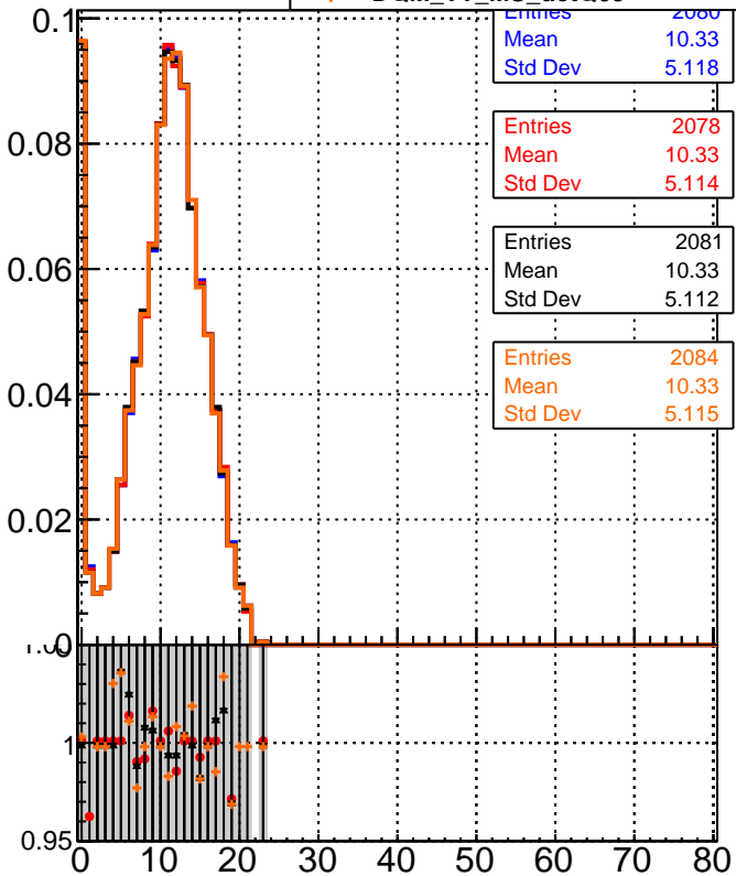
Legend for the bottom row plots: — DQM_TT_MS — DQM_TT_MS_detQ — DQM_TT_MS-detQ1 — DQM_TT_MS_detQ09
