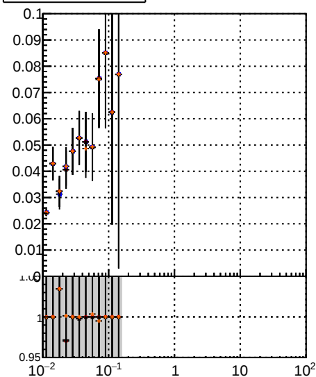
Fake rate vs \sqrt{s} —●— \sqrt{s} det0 —●— \sqrt{s} det01 —●— \sqrt{s} det09
