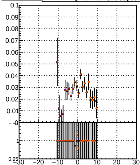
Fake rate vs \sqrt{s} —●— \sqrt{s} det0 —●— \sqrt{s} det01 —●— \sqrt{s} det09
