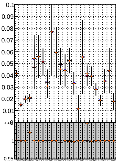
Fake rate vs. BSM \chi^2 MS \chi^2 data \chi^2 BSM \chi^2 MS \chi^2 data \chi^2
