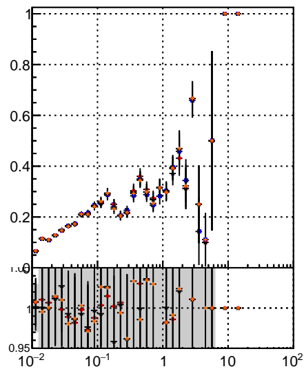
Fake rate vs \sqrt{s} —■— DQM TT MS detQ —●— DQM TT MS detQ1 —▲— DQM TT MS detQ9
