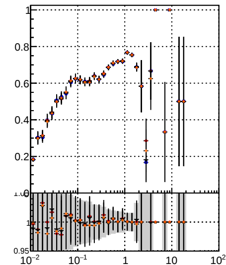
Fake rate vs \nu DOM TT MS det0 DOM TT MS det01 DOM TT MS det09 DOM TT MS det0 DOM TT MS det01 DOM TT MS det09
