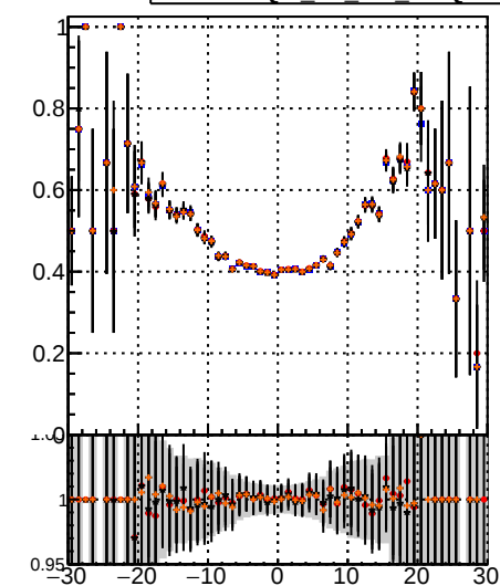
Fake rate vs \nu DQM TT MS det0 DQM TT MS det01 DQM TT MS det09
