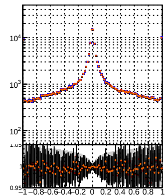
N of reco track vs dxy(PV) MS-det09 MS-det01 MS-det09
