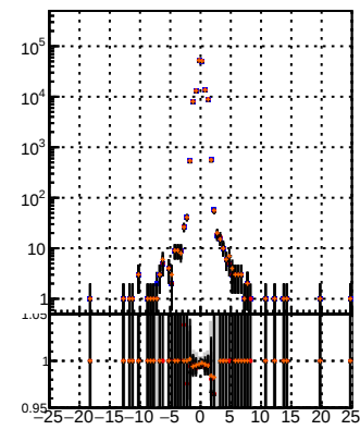
N of reco track vs dxy(PV) MS-det09 MS-det01 MS-det09
