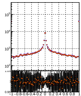
—●— DQM TT MS-det01 —●— DQM TT MS-det09 —●— DQM TT MS-det01 —●— DQM TT MS-det09
