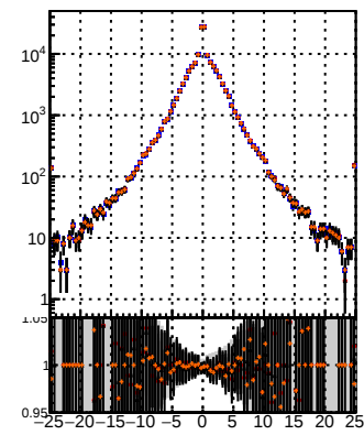
—●— DQM TT MS-det01 —●— DQM TT MS-det09 —●— DQM TT MS-det01 —●— DQM TT MS-det09
