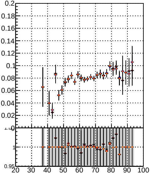
Fakerrate vs PU
