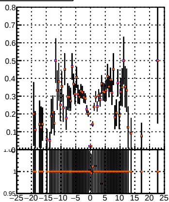
Efficiency DQM_TT_MS DQM_TT_MS_detQ DQM_TT_MS_detQ-dpdq DQM_TT_MS_detQ-chi2
