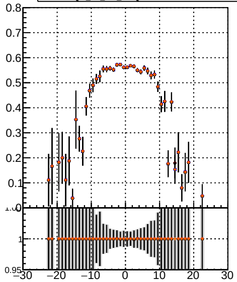
Efficiency vs. sim PV z — DQM TT MS — DQM TT MS detQ — DQM TT MS detQ-dpdq — DQM TT MS detQ-chi2
