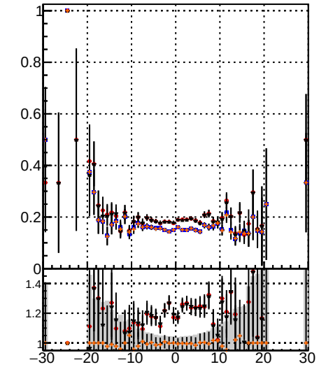
Fake rate vs \sqrt{s} BQM TT MS det0 dndq det0-chiz BQM TT MS det0 dndq det0-chiz
