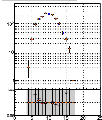
\chi^2
