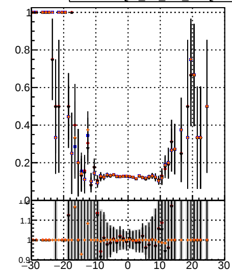
Legend: - \text{BQM} \rightarrow \text{TT} \rightarrow \text{MS} \rightarrow \text{det0} - \text{BQM} \rightarrow \text{TT} \rightarrow \text{MS} \rightarrow \text{det0-dpdq} - \text{BQM} \rightarrow \text{TT} \rightarrow \text{MS} \rightarrow \text{det0-chiz}
