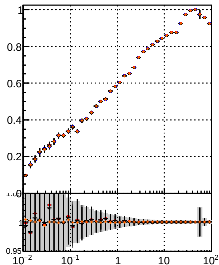
Fake rate vs \sqrt{s} DQM TT MS det0 dndq DQM TT MS det0-chiz
