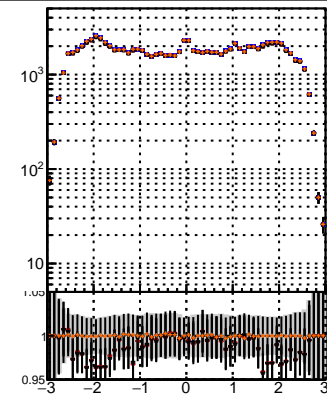
etQ etQ-dpdq etQ-chi2
