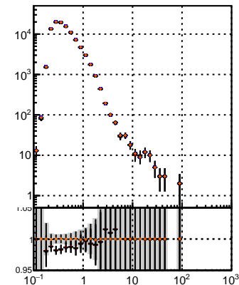
etQ etQ-dpdq etQ-chi2
