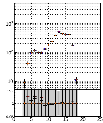
—●— det0-dpda —●— det0-chi2 —●— det0-chi2
