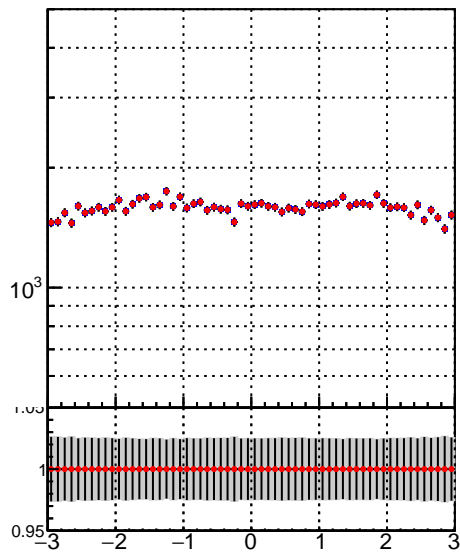
■ Orig/DQM_orig_MS ■ pixelLessOrig/DQM_mod_MS
