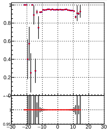
— Orig/DQM_orig_MS —●— pixellLessOrig/DQM_mod_MS
