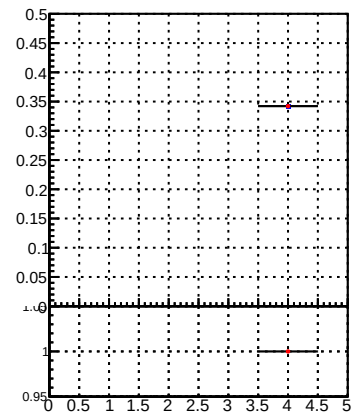
Orig/DQM_orig_MS pixelLessOrig/DQM_mod_MS
