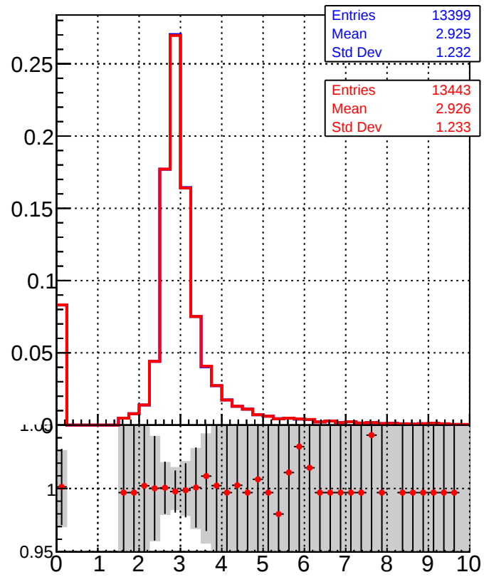
Orig/DQM_orig_MS pixelLessOrig/DQM_mod_MS
