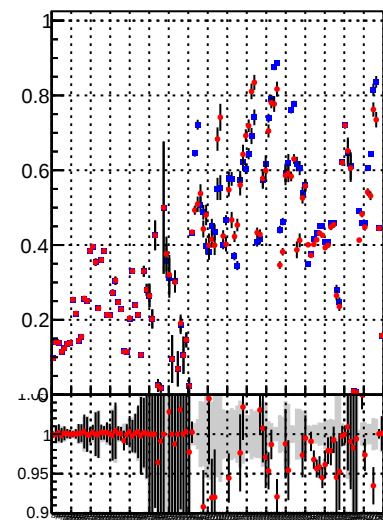
—●— Orig/DQM_orig_MS —●— pixelLessOrig/DQM_mod_MS
