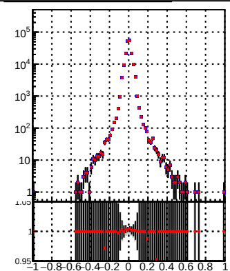
DQM_mod_MS
