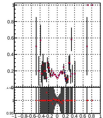
— Orig/DQM_orig_MS — pixelLessOrig/DQM_mod_MS
