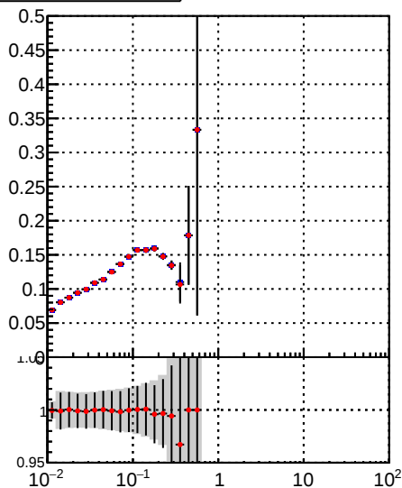
— Orig/DQM_orig_MS — pixelLessOrig/DQM_mod_MS
