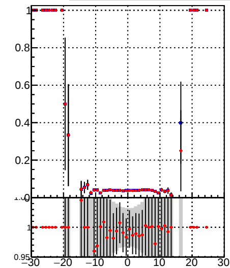
—•— Orig/DQM_orig_MS —•— pixellLessOrig/DQM_mod_MS
