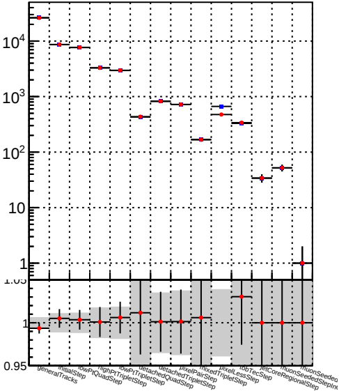
Number — pixelLessOrig/DQM_mod_MS
