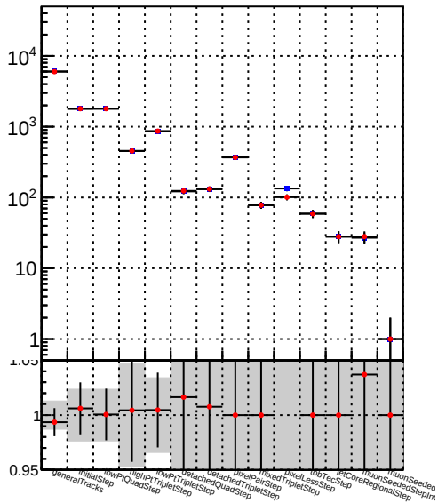
Number — pixelLessOrig/DQM_mod_MS
