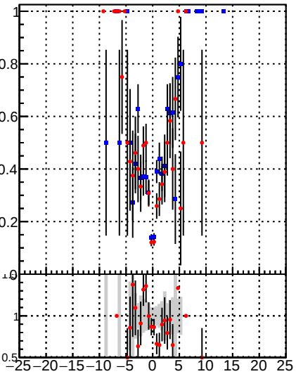
— Orig/DQM_orig_MS — pixelLessOrig/DQM_mod_MS
