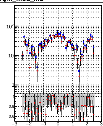
—●— Orig/DQM_orig_MS —●— pixelLessOrig/DQM_mod_MS
