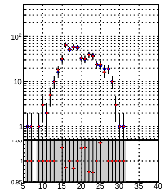
— Orig/DQM_orig_MS — pixelLessOrig/DQM_mod_MS
