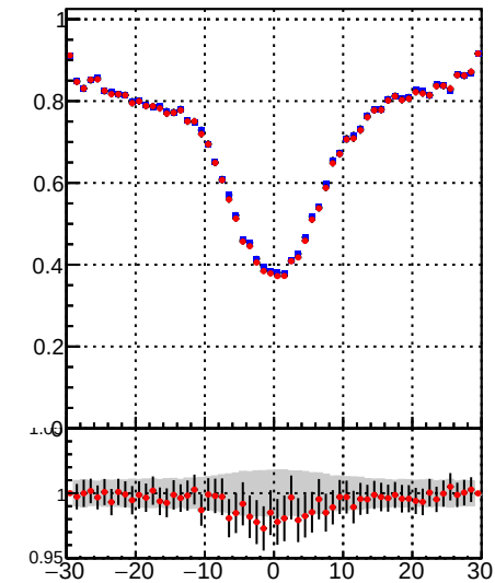
—●— Orig/DQM_orig_MS —●— pixelLessOrig/DQM_mod_MS
