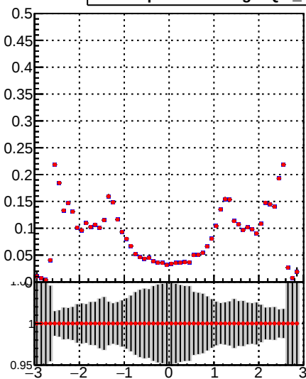
—•— Orig/DQM_orig_MS —•— pixelLessOrig/DQM_mod_MS
