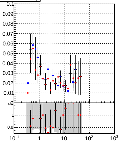
Orig/DQM_orig_MS pixelLessOrig/DQM_mod_MS
