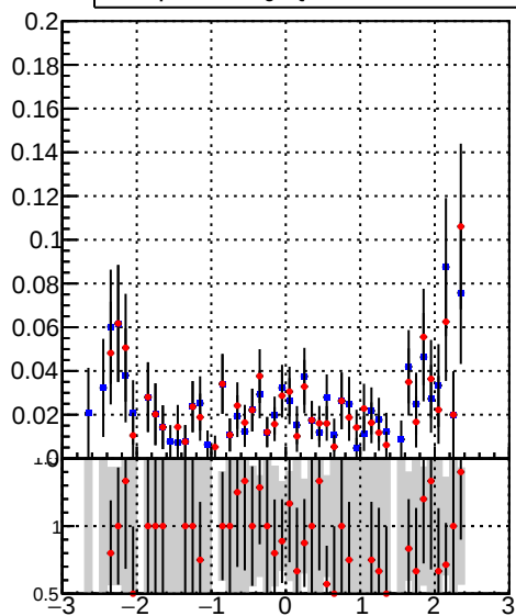
Orig/DQM_orig_MS pixelLessOrig/DQM_mod_MS
